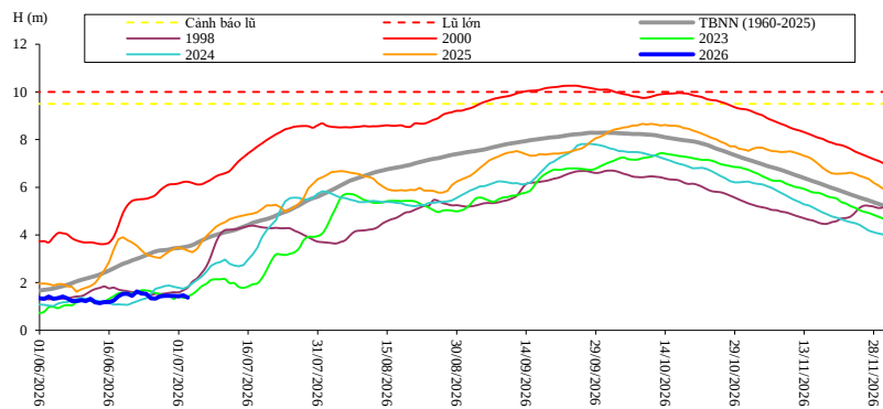
Dòng chảy lúc 7 giờ sáng từ 01/06/2026-03/07/2026 tại trạm Prek Kdam
