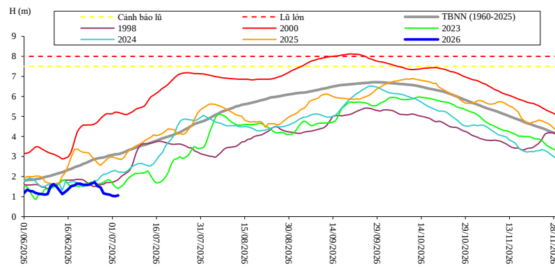
Dòng chảy lúc 7 giờ sáng từ 01/06/2026-03/07/2026 tại trạm Neak Luong
