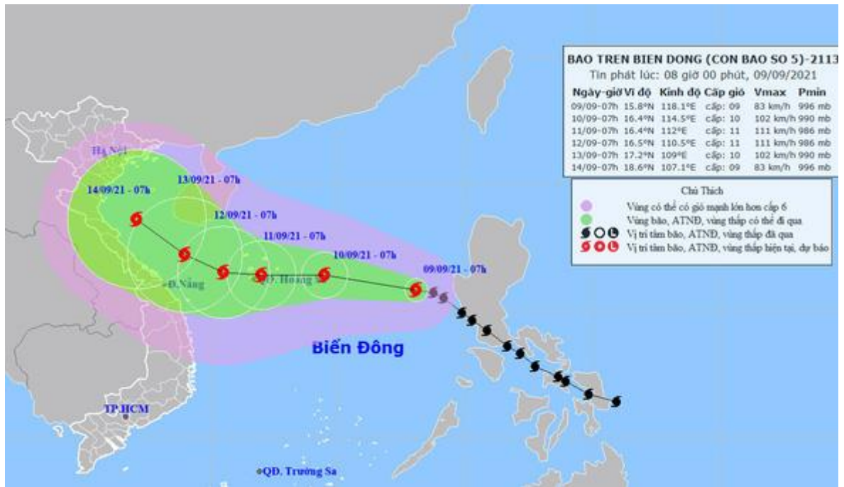
Hình 1. Đường đi dự báo của cơn bão số 5
