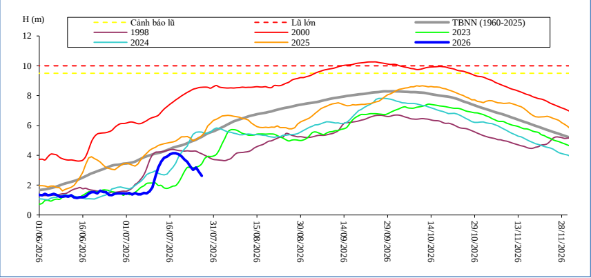
Dòng chảy lúc 7 giờ sáng từ 01/06/2026-27/07/2026 tại trạm Prek Kdam
