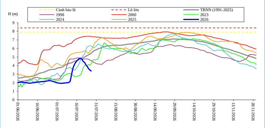
Dòng chảy lúc 7 giờ sáng từ 01/06/2026-27/07/2026 tại trạm Koh Khel
