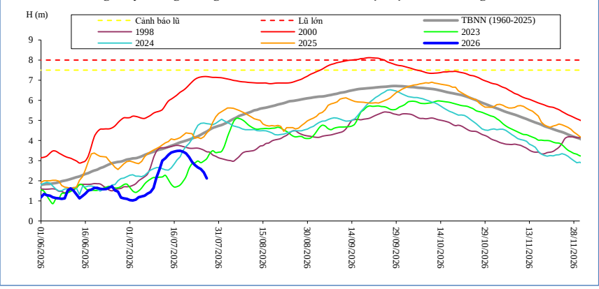
Dòng chảy lúc 7 giờ sáng từ 01/06/2026-27/07/2026 tại trạm Neak Luong
